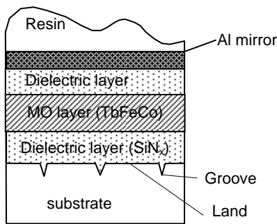
図 7 光磁気ディスクの構造
