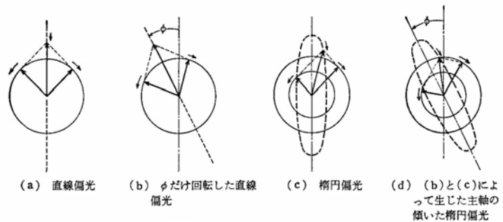
図 1 旋光性と円二色性の起源
