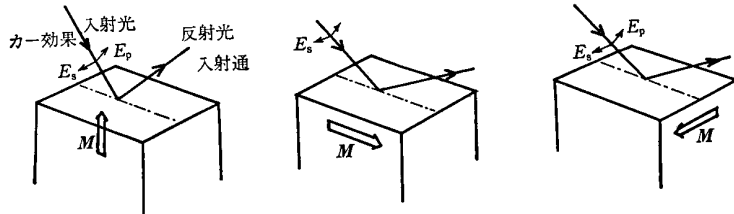
図2 磁気カー効果
